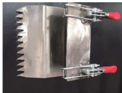
吴炜设计的破袋器
